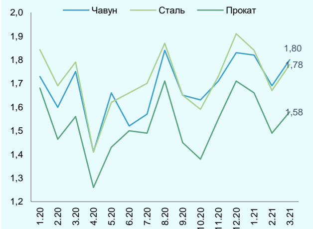
Рис.2.6 Виробництво чавуну, сталі та прокату (дані Укрметалургпром), млн.т
